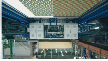
CHROMOJET 76 DPI 工艺印花
